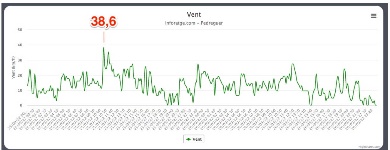
Ráfagas de viento registradas en PEDREGUER el 25 y el 26/09/22 (en km/h) https://inforatge.com/meteo-pedreguer
